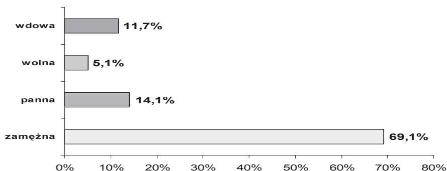
Wykres 4. Status rodzinny respondentek
