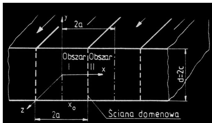
Rys.1. Przekrój modelu domenowego anizotropowej blachy elektrotechnicznej [2]
