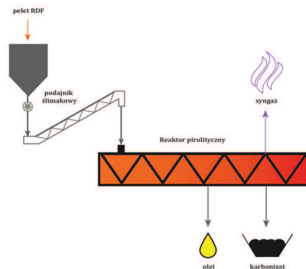
Rysunek 2. Schemat ideowy procesu pirolizy z wykorzystaniem reaktora pirolitycznego ze spiralą grzejną, źródło: materiały własne – Metal Expert Sp. z o.o. Sp. J.
