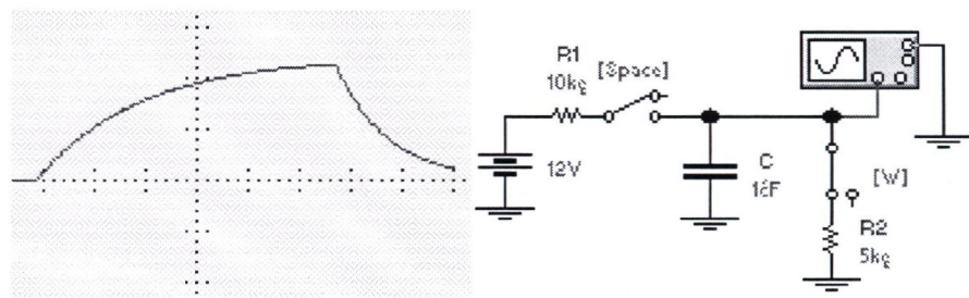
Rys. 4. Badanie stanów nieustalonych w kondensatorze
