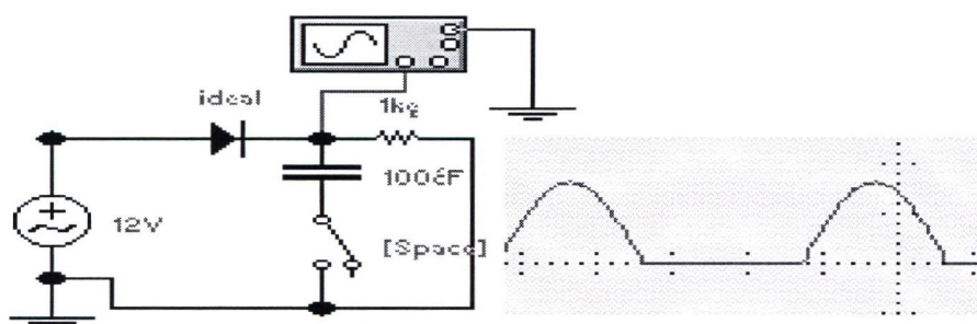
Rys. 6. Prostownik jednopulsowy
