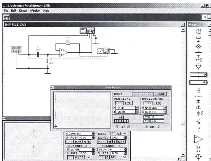
Rys. 1. Zdjęcie przedstawia wygląd programu w części z elektroniki analogowej
